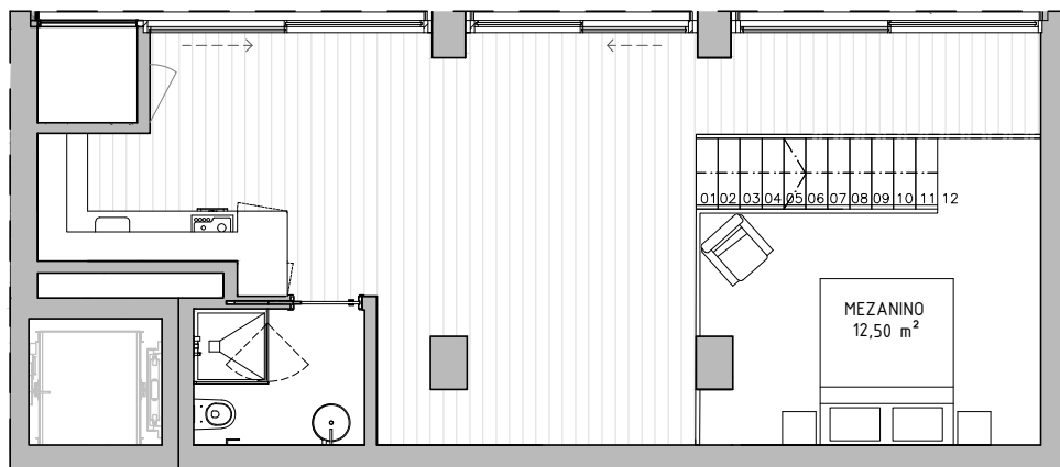
PLANTA MEZANINO
