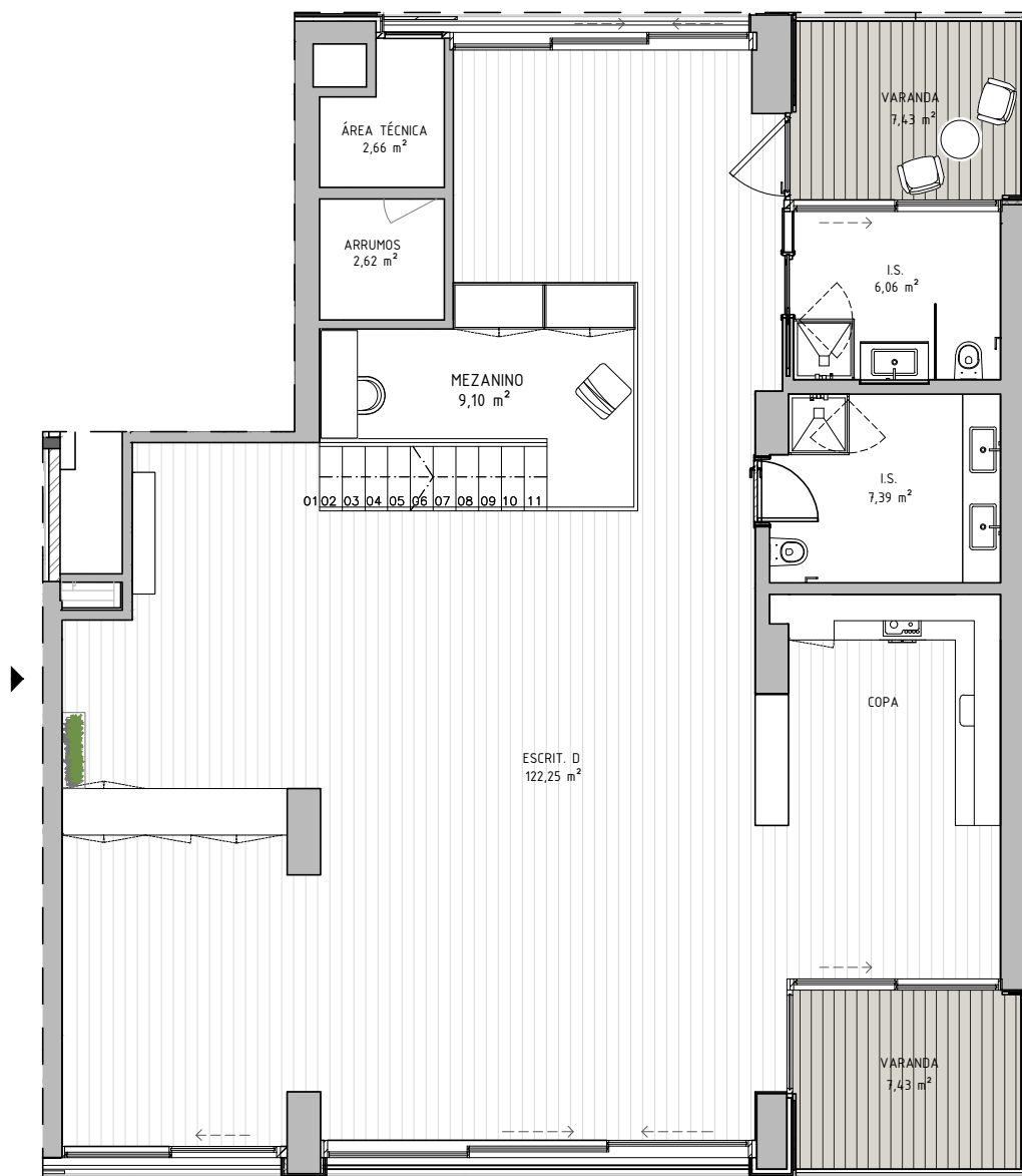
PLANTA MEZANINO
