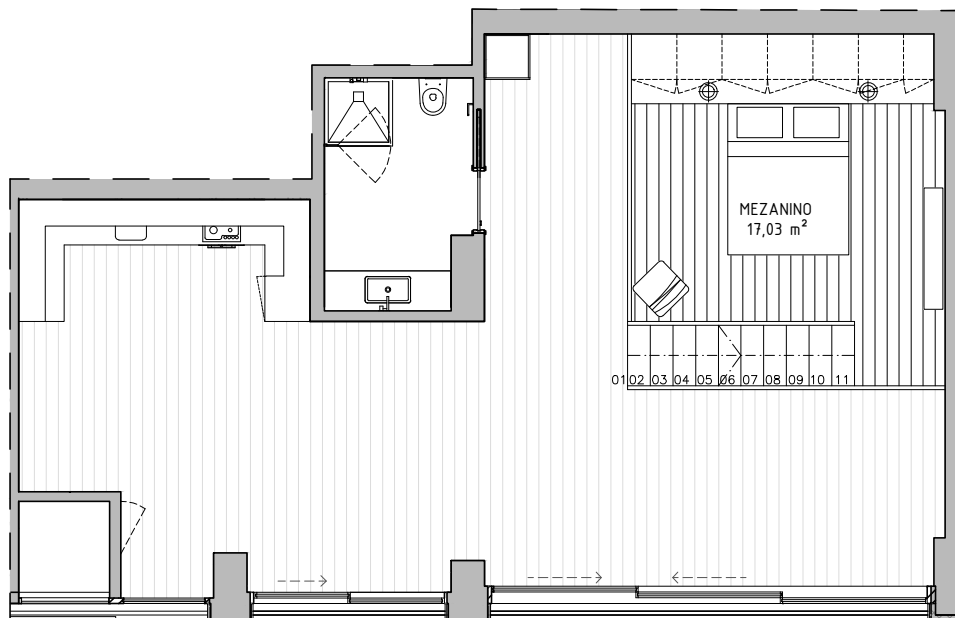
PLANTA MEZANINO
