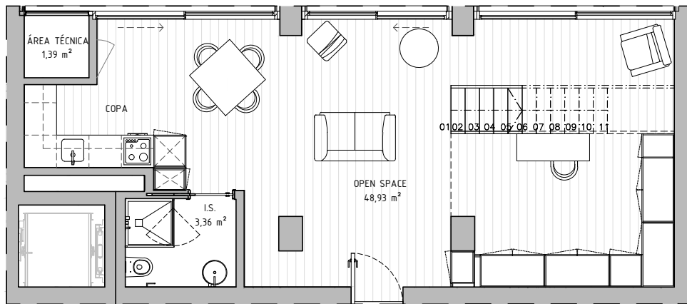
PISO 0
