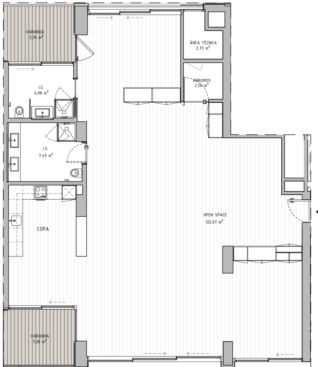
PLANTA
