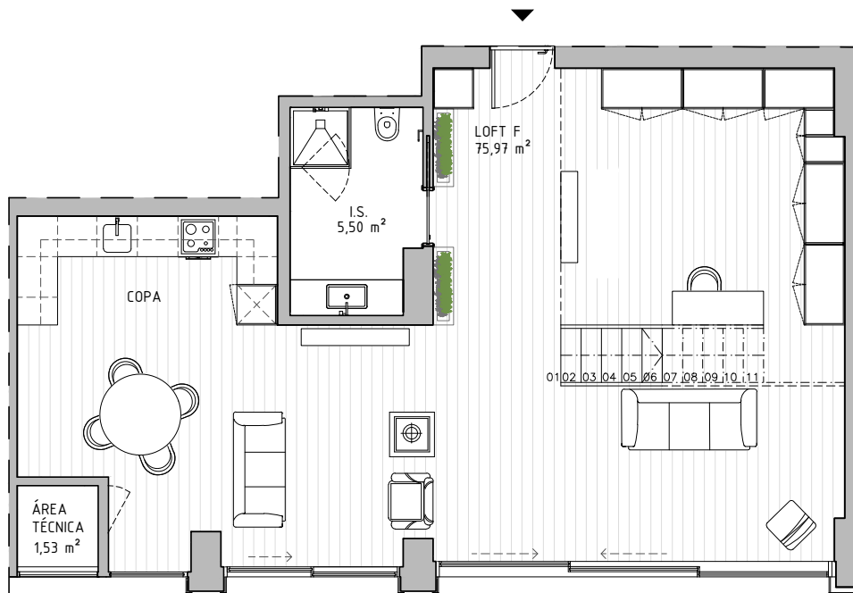
PLANTA
